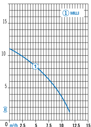
Grindex Milli
