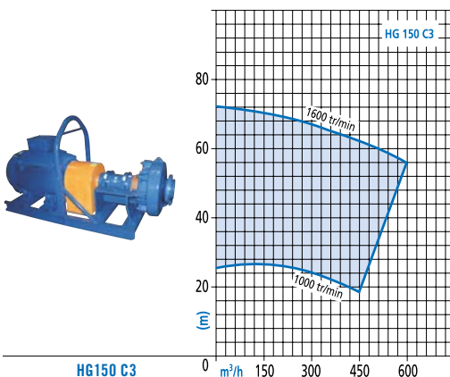
HG150 C3 châssis fixe 20 m de câble électrique. En location, livrée avec : armoire de démarrage à variateur
