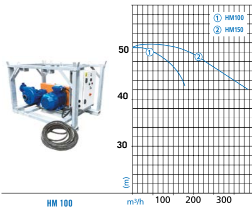
HM100, HM150 chariot fixe, 20 m de câble électrique. En location, livrées avec : armoire de démarrage, sans prise
