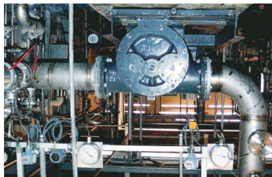
Pompe V180 SPG sur site chimique
