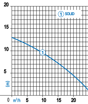
Grindex Solid
