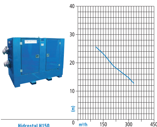
Hidrostral H150
