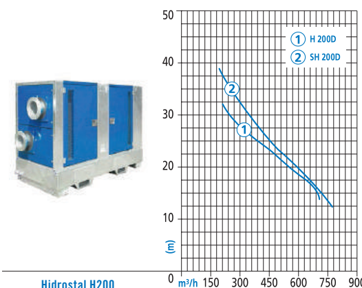
Hidrostral H200
