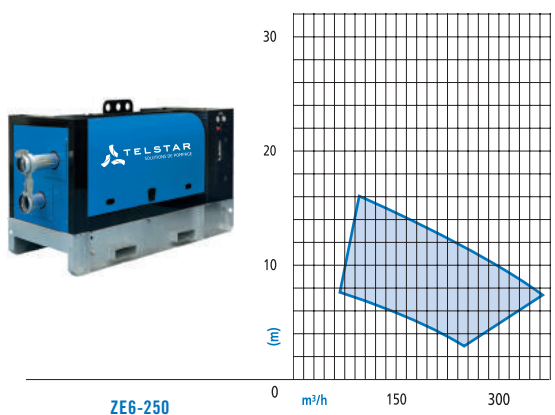
ZE6-250
