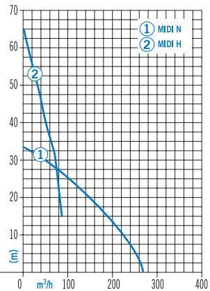
Grindex Midi
