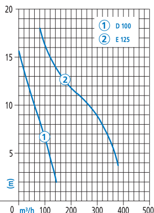
Hidrostral E 125
