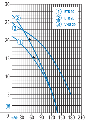
Toyo ETR 10
