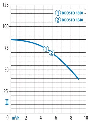
Boosto 1860
